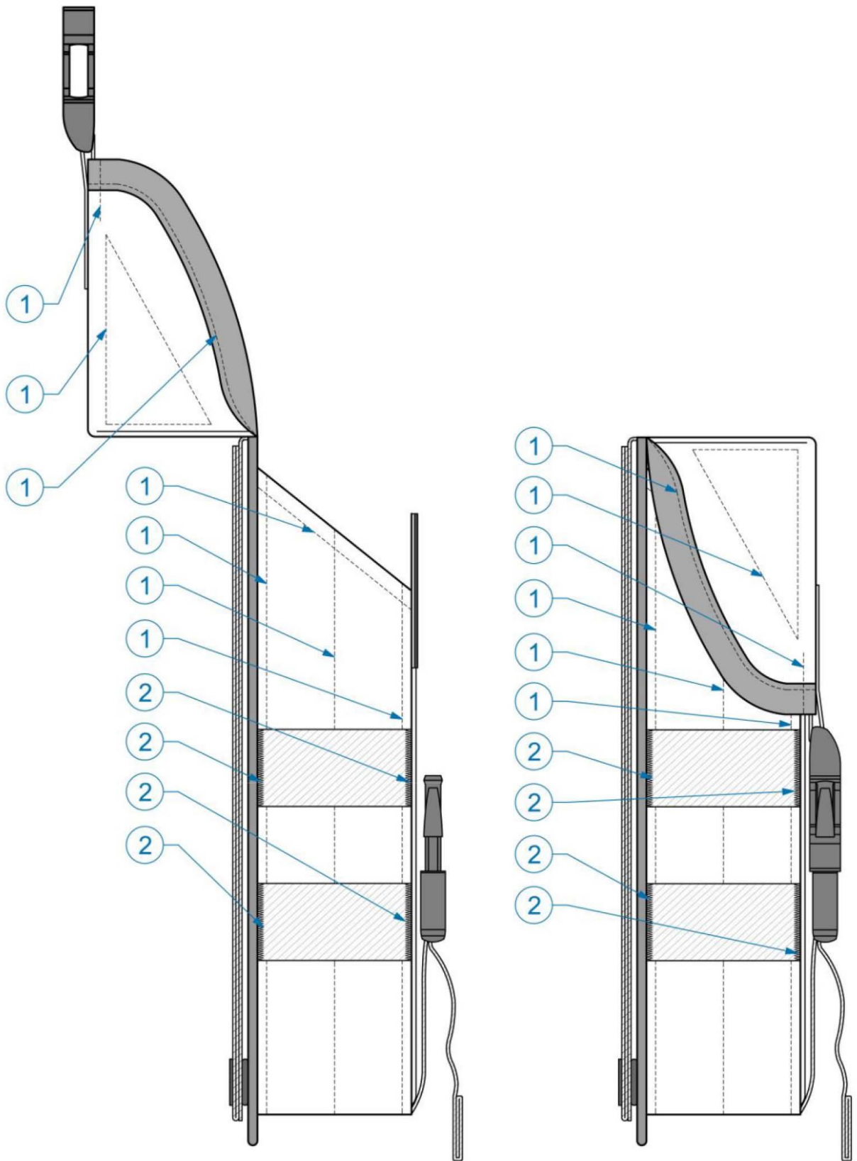
Рисунок Д3.2 — Позначення строчок предмета (вигляд збоку)
