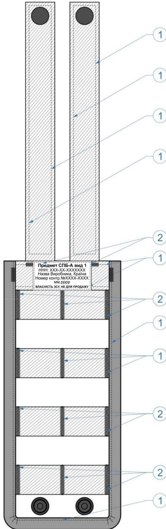
Рисунок Д3.3 — Позначення строчок предмета (вигляд ззаду)
