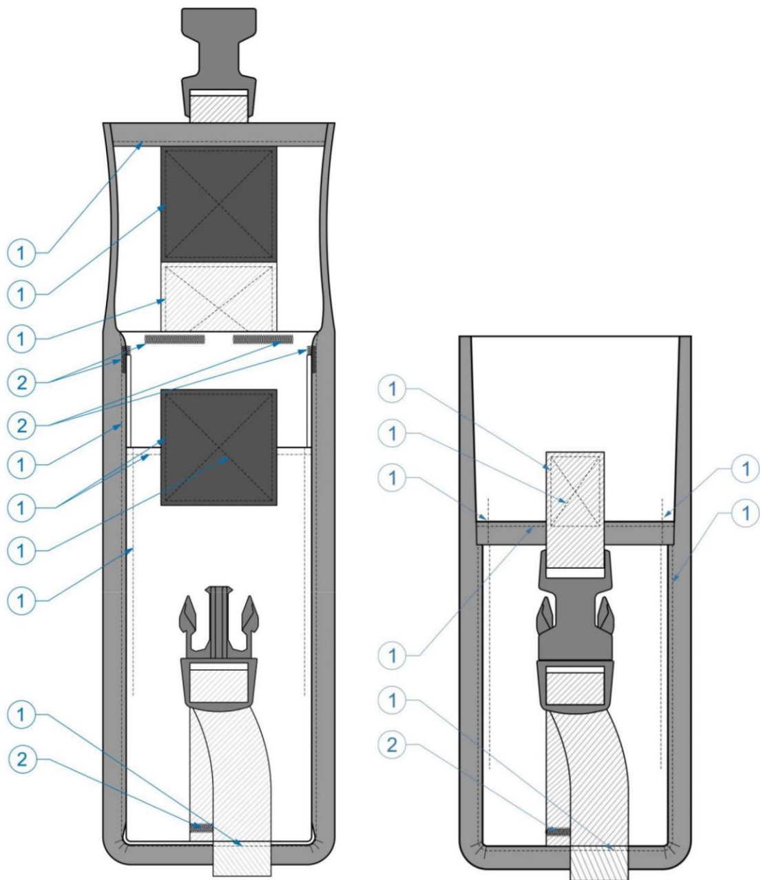
Рисунок ДЗ.1 — Позначення строчок предмета (вигляд спереду)
