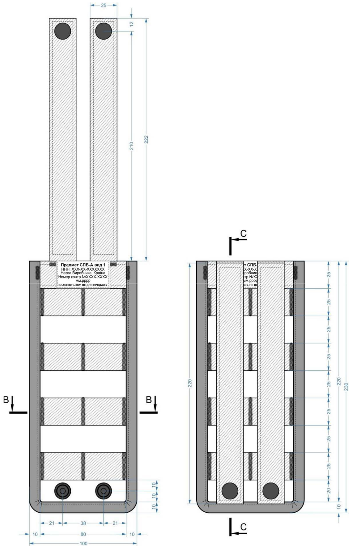
Рисунок Д2.3 – Схематичне зображення предмета із позначенням лінійних вимірів (вигляд ззаду)
