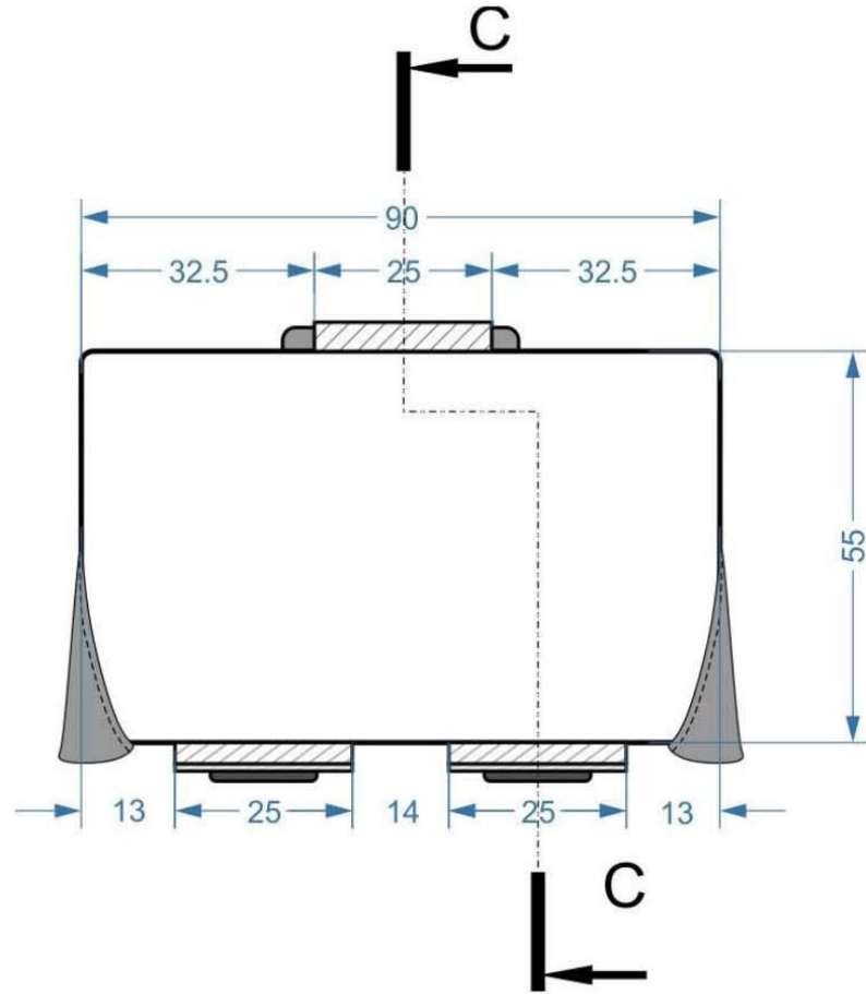
Рисунок Д2.4 – Схематичне зображення предмета із позначенням лінійних вимірів (вигляд зверху)
